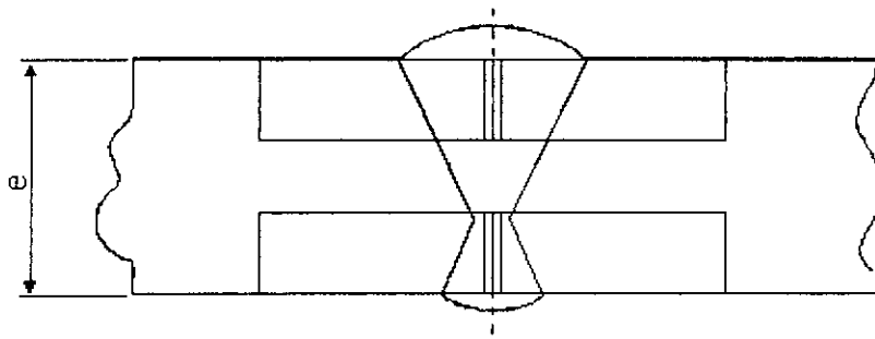
Oś spoiny
